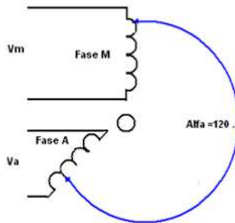
Fig. 7 Máquina monofásica asimétrica.
