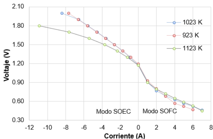
Fig. 2. Curvas de activación de la celda reversible con diferentes temperaturas de los gases reaccionantes.
