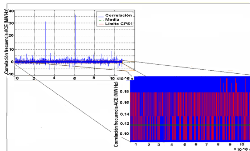
Fig. 2. Verificación criterio CPS1 con \varepsilon_1 = 30\text{mHz}
