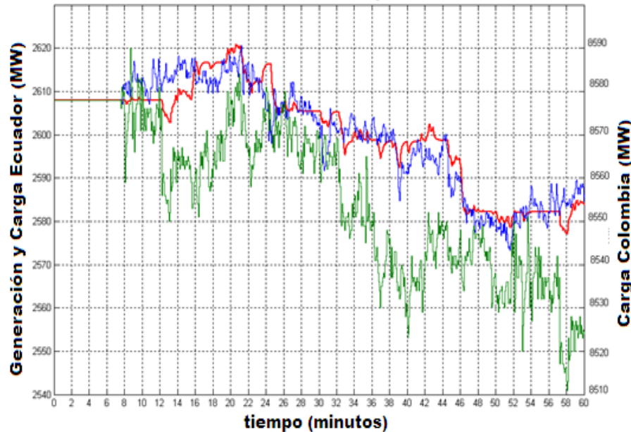
Fig. 6. Gráfico de la Generación del Ecuador la carga del Ecuador y la carga de Colombia versus tiempo. El eje izquierdo de las ordenadas contiene la escala de la generación y de la carga del Ecuador. El eje derecho de las ordenadas contiene la escala de la carga de Colombia.
