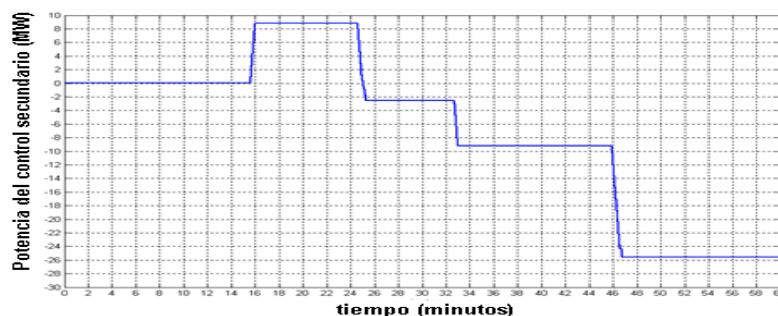
Fig. 11. Comportamiento del control secundario de la frecuencia en el SNI del Ecuador en el periodo de demanda punta en un día laborable típico.
