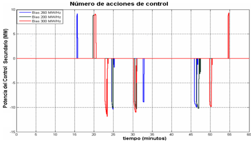
Fig. 7. Número de acciones de control en régimen de máxima generación para las diferentes posibilidades de ajuste del factor BIAS. Azul: 250 MW/Hz, Verde: 200 MW/Hz, Rojo: 300 MW/Hz.
