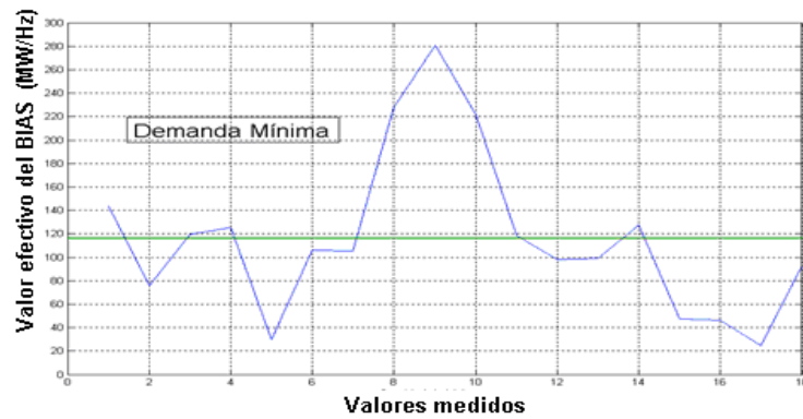
Fig. 9. Cálculo del estatismo efectivo del SNI del Ecuador en demanda mínima.
