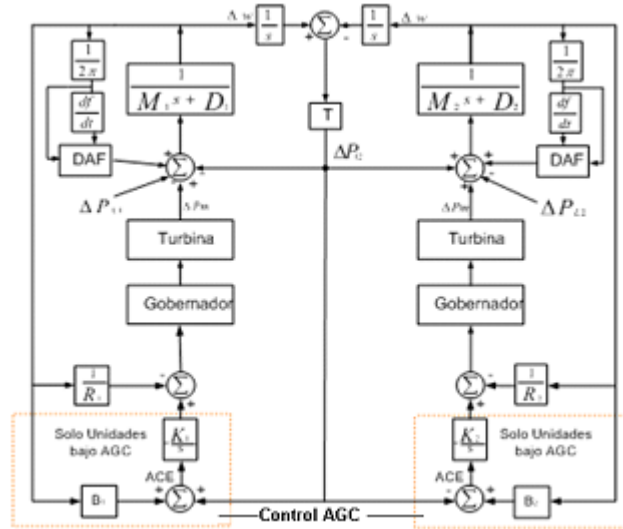
Fig. 1. Esquema Concentrado Equivalente para el estudio del control de la frecuencia.
