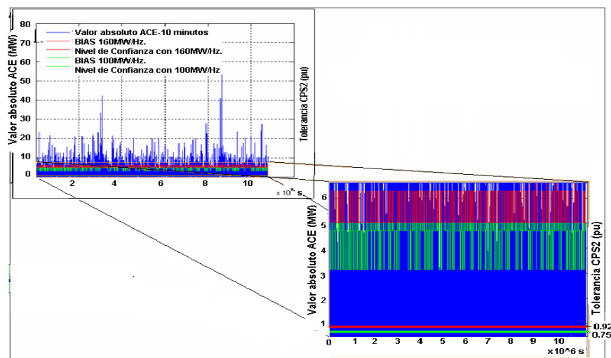
Fig. 4. Verificación criterio CPS2 aumentando el valor mínimo del BIAS asignado en el sistema eléctrico del Ecuador.
