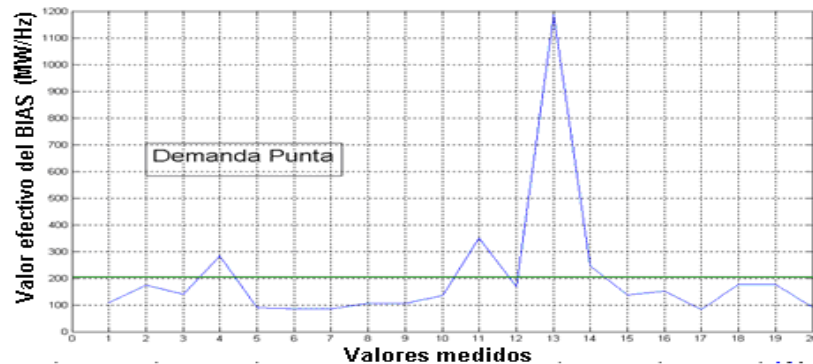
Fig. 10. Cálculo del estatismo efectivo del SNI del Ecuador en demanda máxima.
