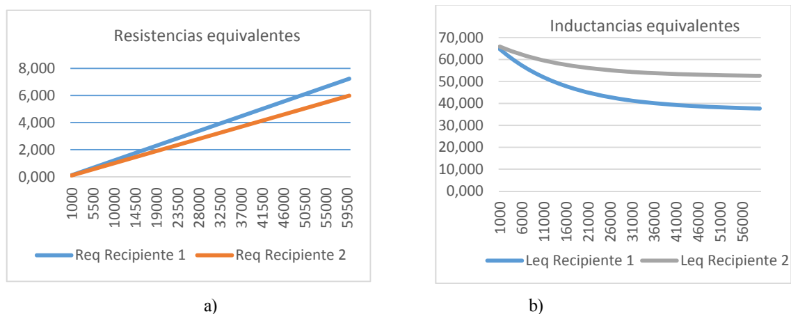
Fig. 3. Parámetros de la impedancia equivalente estimada. a) Resistencia equivalente. b) Inductancia equivalente.
