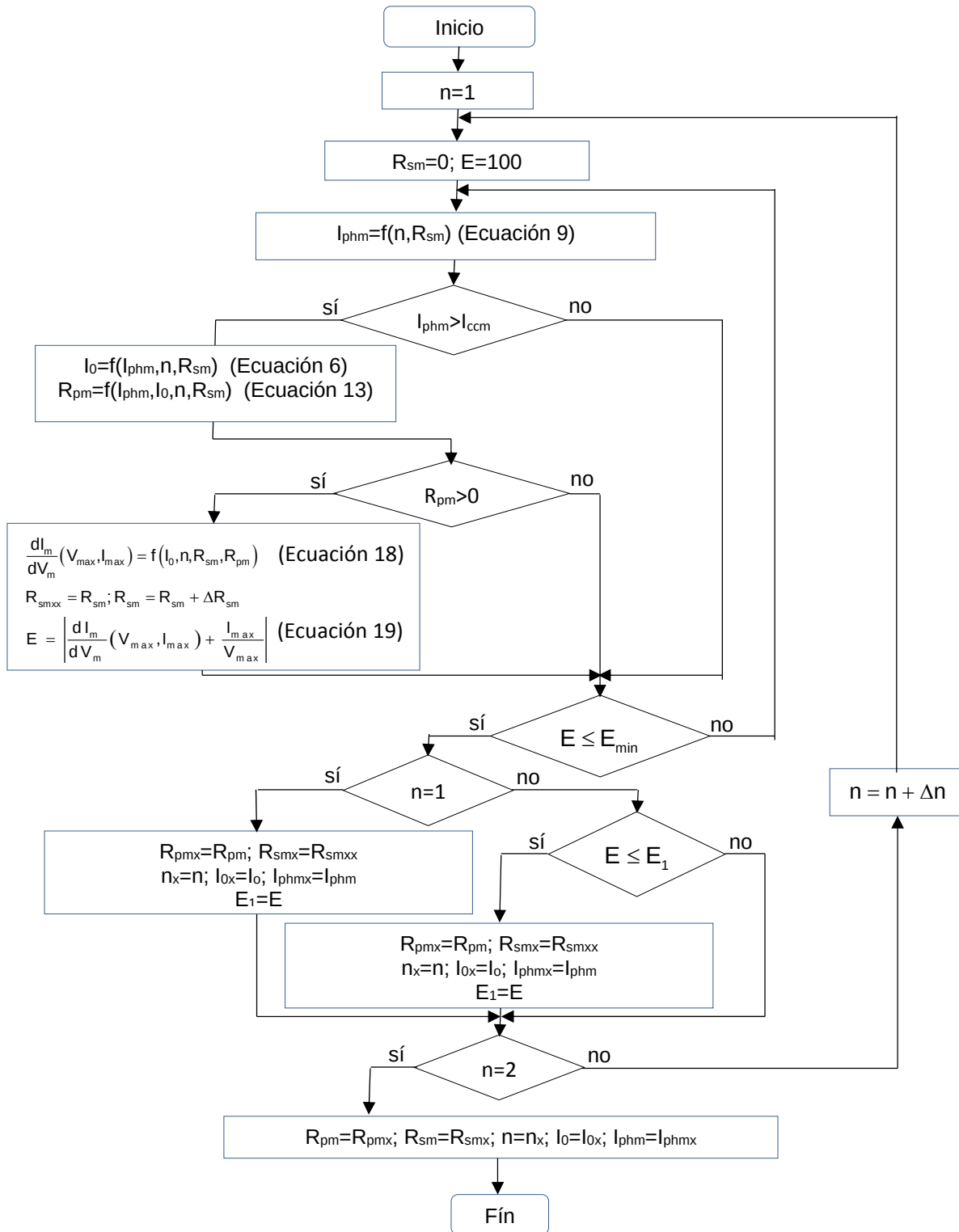
Fig. 4. Algoritmo de cálculo de los cinco parámetros del circuito equivalente.
