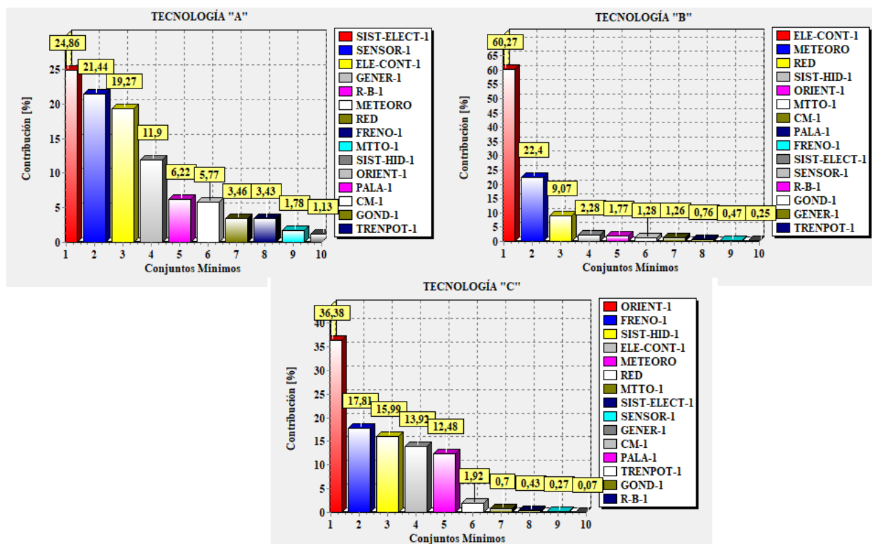
Fig. 8. Distribución de fallos por máquina para tecnologías A, B y C.
