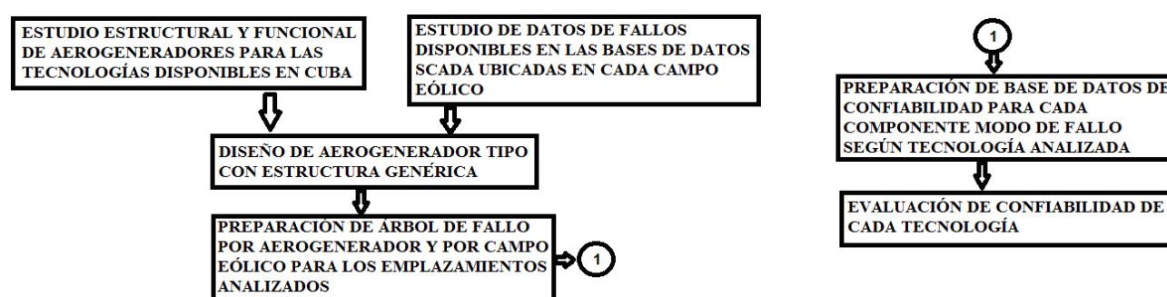
Fig. 4. Algoritmo de estudio de confiabilidad tecnológica de campos eólicos [7].
