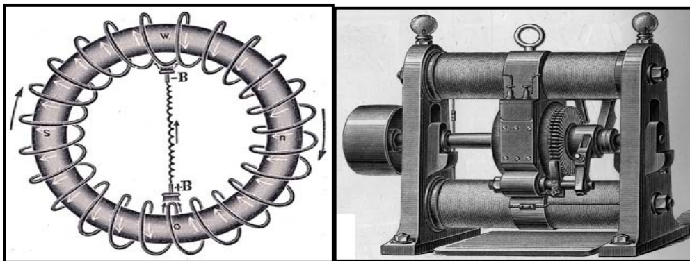
Fig. 2. Izquierda: Anillo de Gramme, primer conmutador mecánico para máquinas de corriente directa. Derecha: Motor de Gramme ampliando el empleo exitoso de la tecnología constructiva de Werner Siemens.
