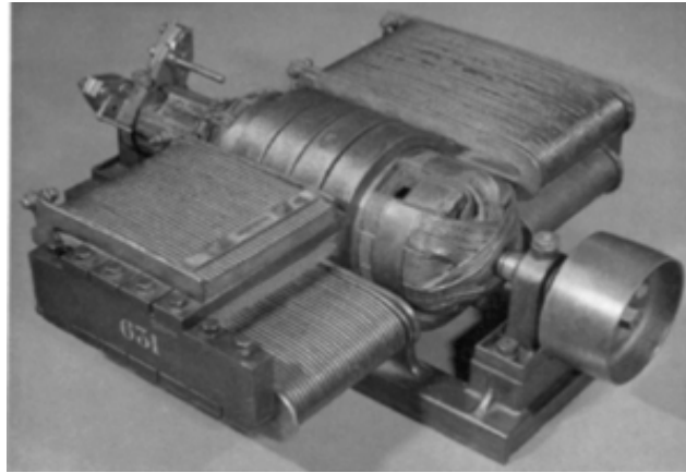
Fig. 3. “Tambor de Siemens” (1872) conservado en el Museo de Ciencias de Londres.
