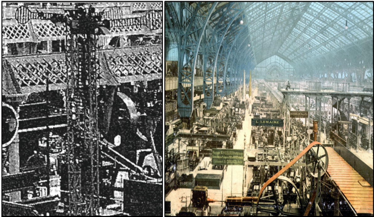
Fig. 12. Izquierda: Montaje con una grúa torre (precursor de grúa torre actual) de un pórtico eléctrico en la exposición, se montaron piezas con un peso de 48 toneladas. Derecha: Interior de la Galería de Máquinas, observar numerosos accionamientos por correa con motores eléctricos.
