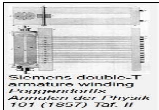
Fig. 1. Generador Siemens con armadura cuyos enrollados doble T vienen por primera vez sumidos en ranuras, funcionaba de forma manual produciendo pulsos.
