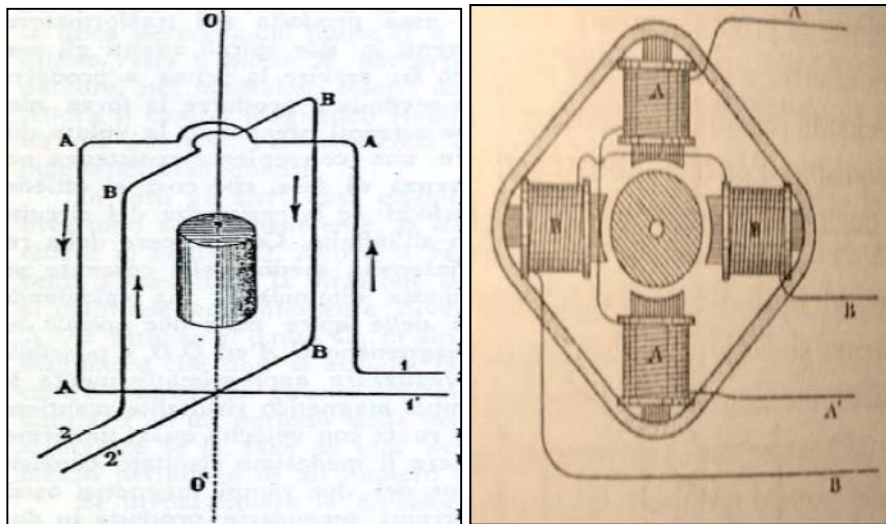
Fig. 4. Primer motor de inducción (bifásico) diseñado por el científico italiano Ferraris.
