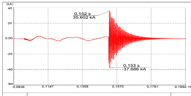
Fig 11. Corriente de descarga que pasa por el neutro del banco de condensadores para un cortocircuito trifásico cuando la tensión es máxima en la fase A.
