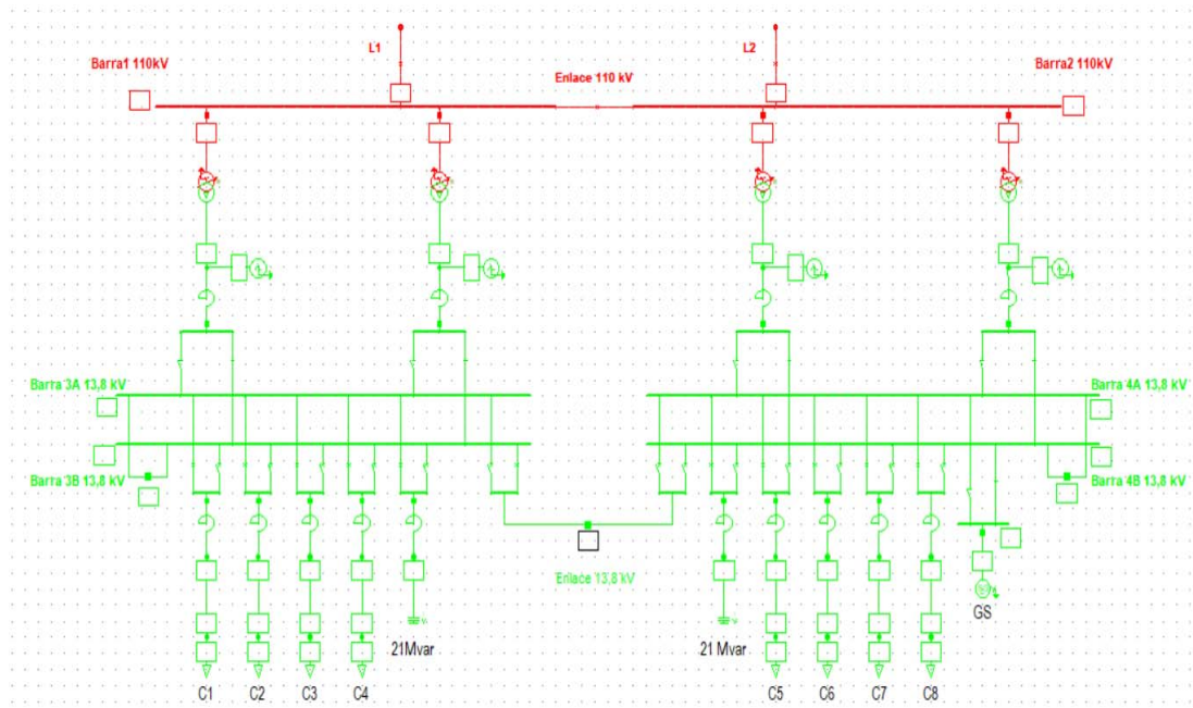
Fig 1. Esquema unifilar simplificado de la subestación Tallapiedra.
