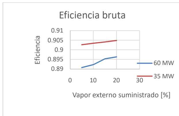
Fig. 2. Eficiencia bruta del generador de vapor en régimen complejo
