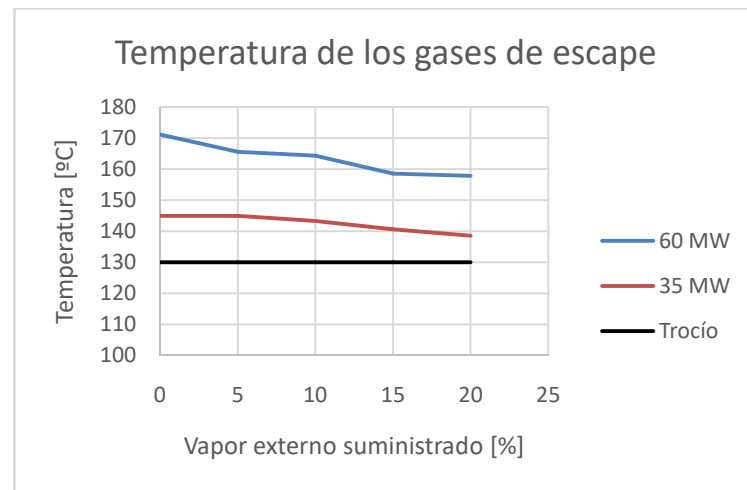
Fig. 5. Temperatura de gases de escape en régimen complejo
