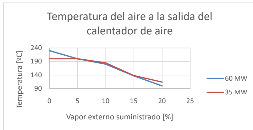
Fig. 6. Temperatura del aire a la salida de calentador de aire en régimen complejo
