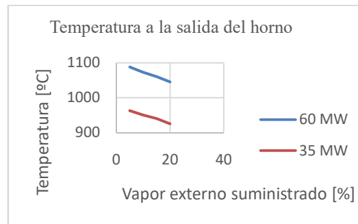
Fig. 4. Temperaturas de salida del horno para cada uno de los regímenes
